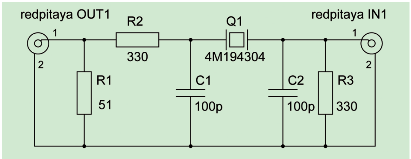
Caption: Figur 1. Diagram af måleopstillingen.
